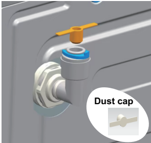
Step 1) Remove the dust cap
